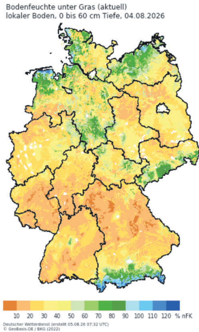
Bodenfeuchte in 0 bis 60 cm Tiefe unter Gras am 4. August. Bei weniger als 30 Prozent nutzbarer Feldkapazität stehen Pflanzen unter deutlichem Trockenstress. Grafik: DWD
